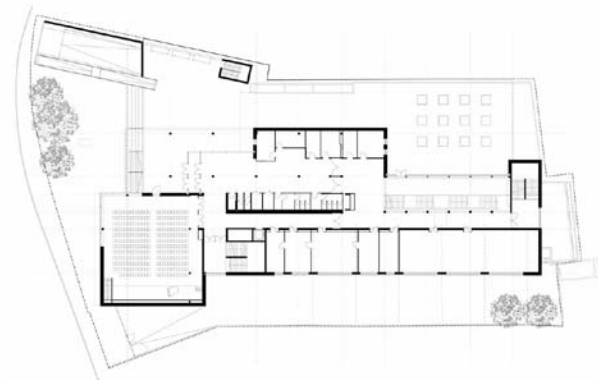
Grundriss EG, überarbeiteter NeuEntwurf (Neubau) Foto: Karl + Probst
